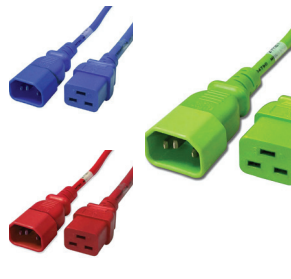
IEC60320 C14 to C19 14AWG SJT Color
